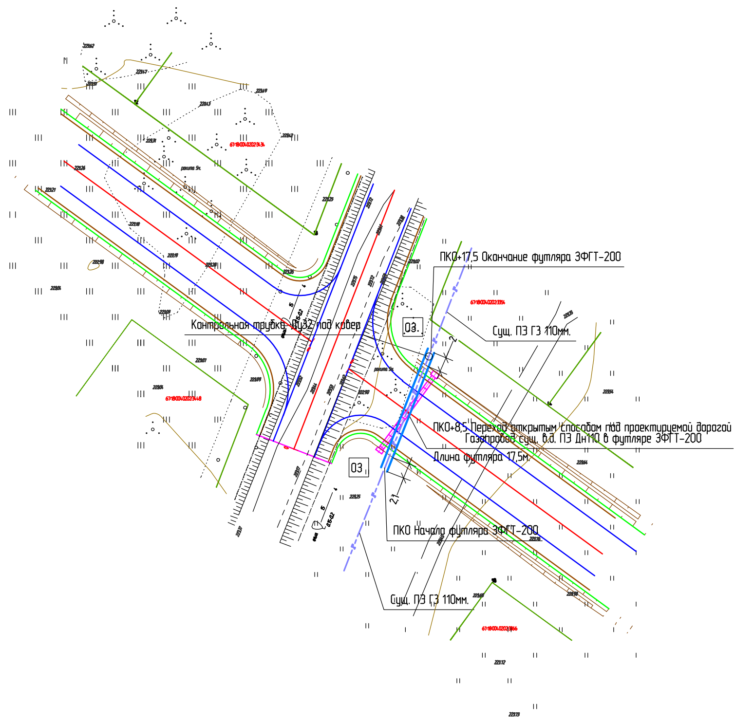
План защиты газопровода М 1:500
